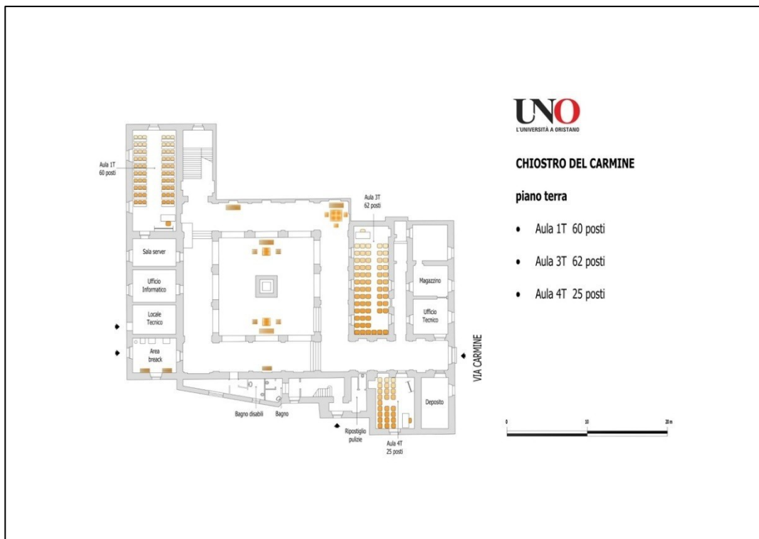
Fig. 1 – Chiostro del Carmine – piano terra
