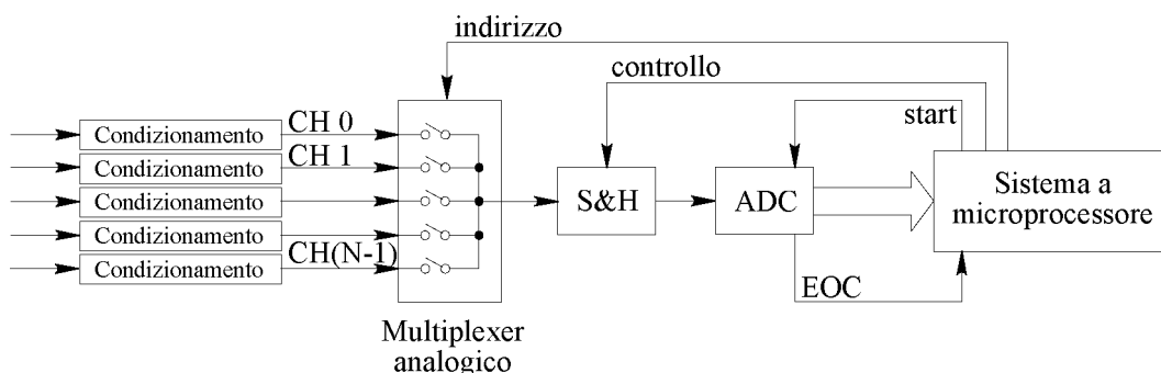
Fig.1.2 - Sistema multicanale con multiplexer.
