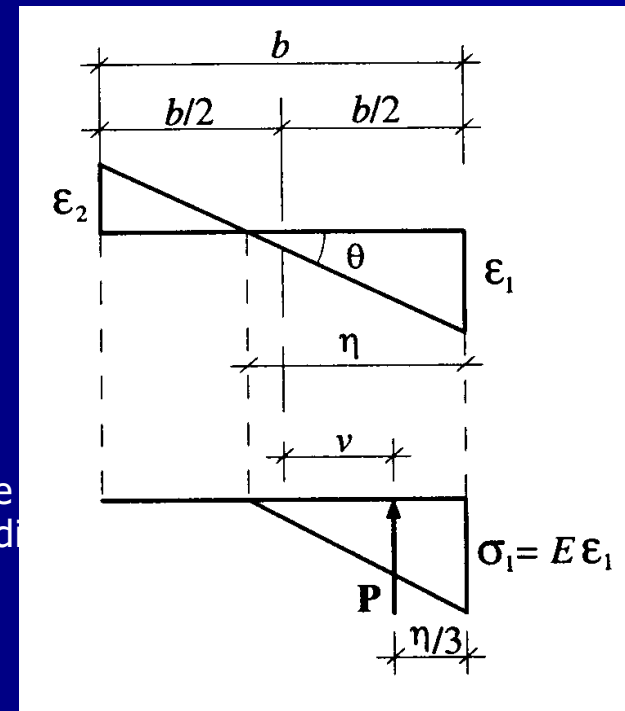
Diagramma delle deformazioni e degli sforzi per un concio con sezione parzializzata.
