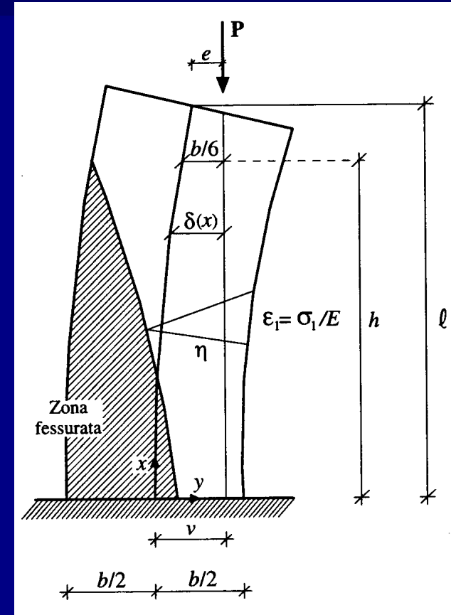
Modello continuo di un pilastro in materiale NRT, nel quale tutti i conci sono deformabili.
