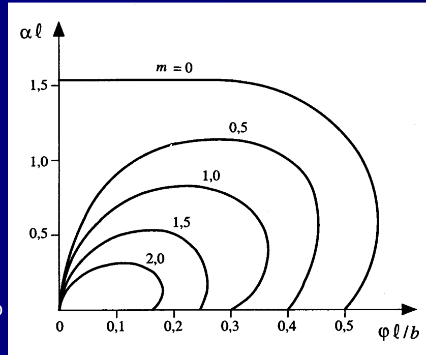
Curve adimensionali carico-rotazione in sommità per il modello continuo del pilastro in muratura NRT.
