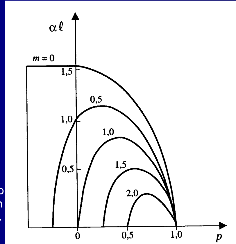
Curve carico-spostamento (in forma adimensionalizzata) per il modello continuo del pilastro in muratura NRT.
