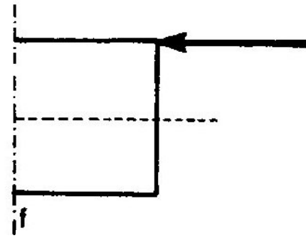
f Pressoflessione: limite di concentrazione sforzi sulla fibra esterna
