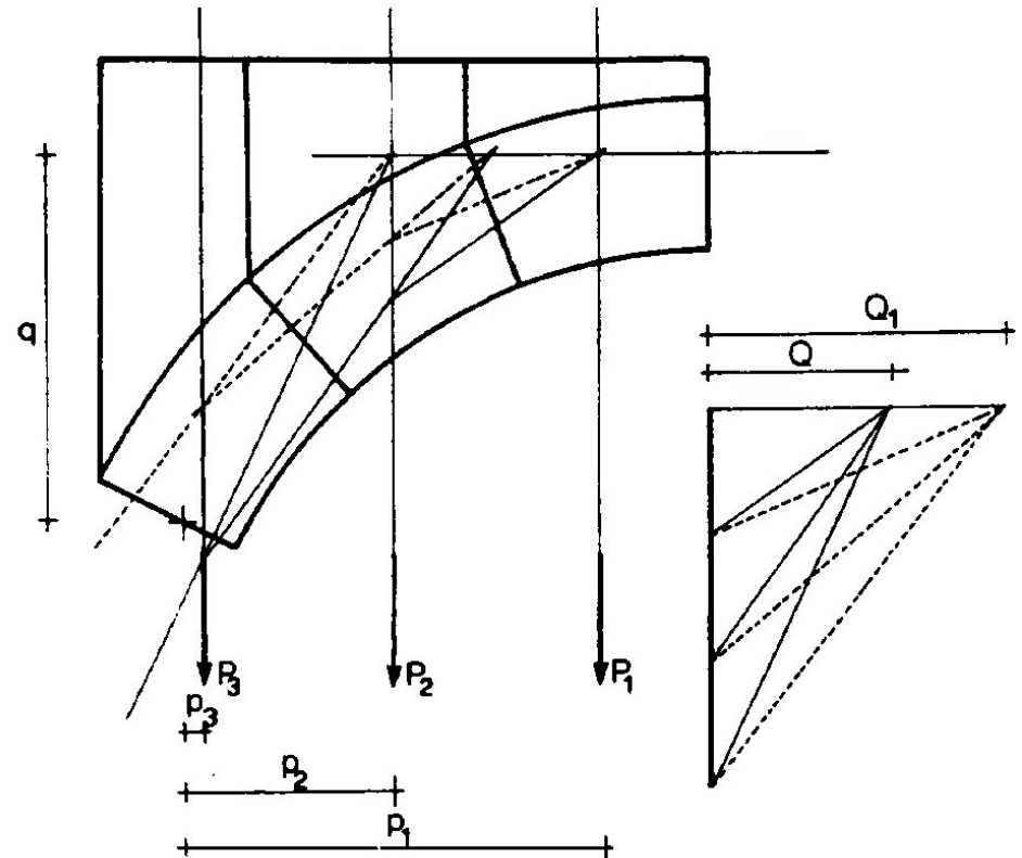
Curve delle pressioni passanti per uno stesso punto e retta di Culmann. (Immagine tratta da Pozzi, op. cit. )
