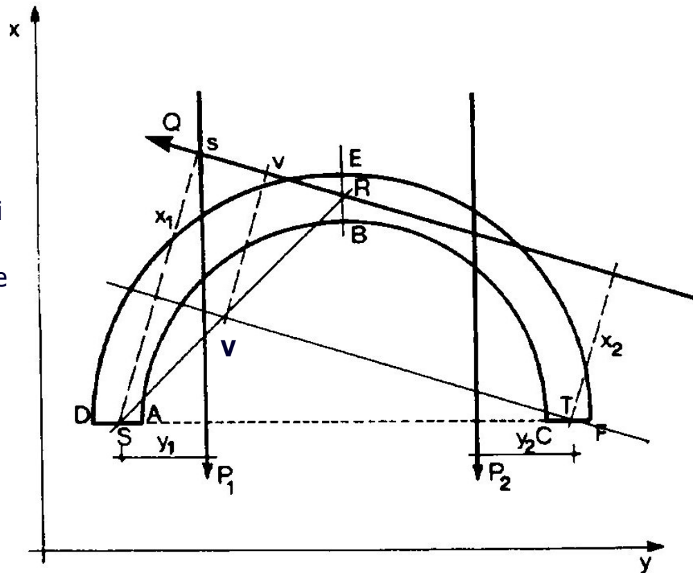
Curva delle pressioni passante per 3 punti. (Immagine tratta da Pozzi, op. cit. )
