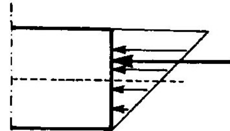
c Pressoflessione con risultante al bordo del nocciolo
