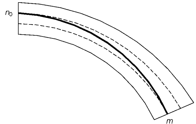
Il canale statico individuato dal terzo medio delle sezioni.
