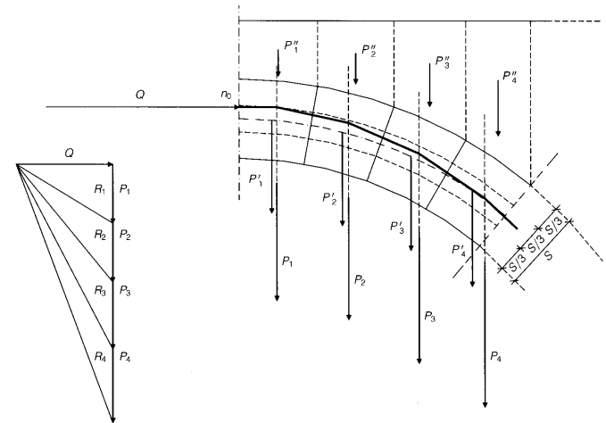
Costruzione della curva delle pressioni per un arco.
