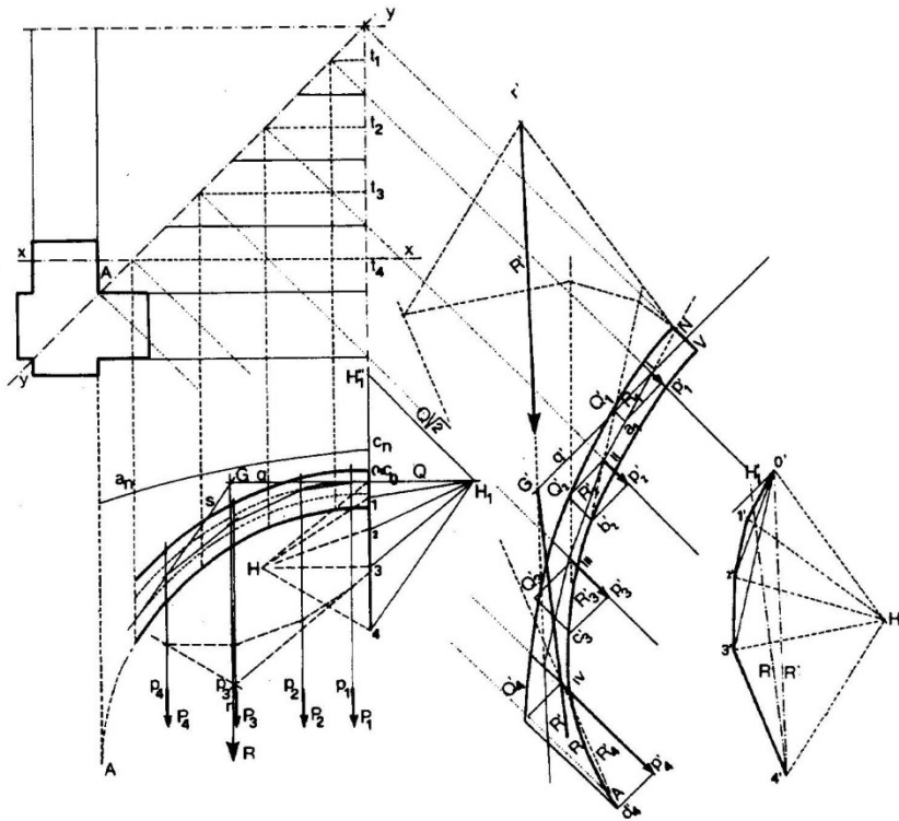
Estensione del procedimento di Mery alla verifica di una volta a crociera (Immagine tratta da Pozzi, op. cit. )
