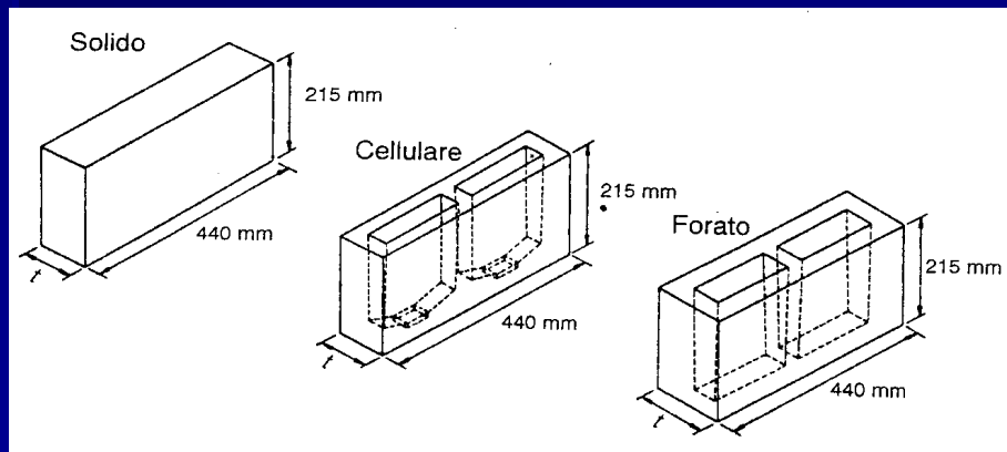
Blocchi in calcestruzzo. (Immagine tratta da Hendry et al. , op. cit. )
