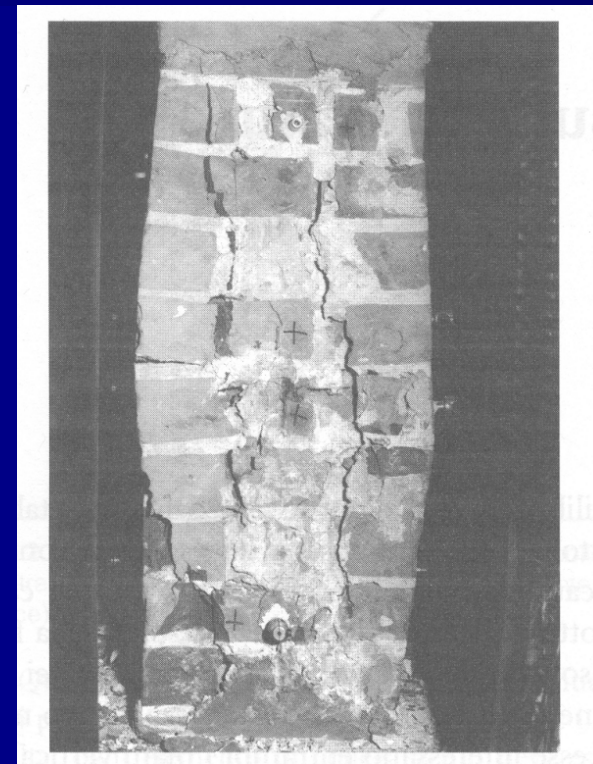
Fessurazioni in un elemento di muratura compresso e prossimo alla rottura.
