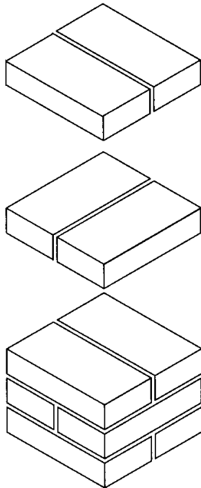
Pilastro in muratura a due teste
