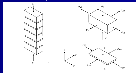
Stato di sforzo nella malta e nel laterizio. (Immagini tratte da Carbone et al. , op. cit. )
