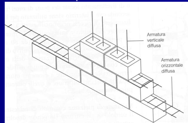
Muratura armata con armatura diffusa. (Immagini tratte da Carbone et al. , op. cit. )
