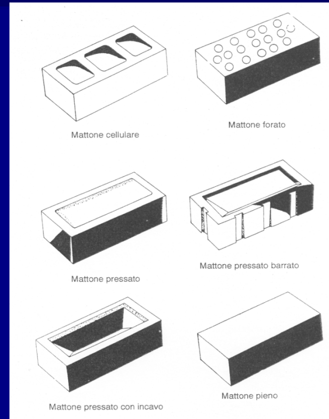
Tipi di mattone standard. (Immagine tratta da Hendry et al. , op. cit. )
