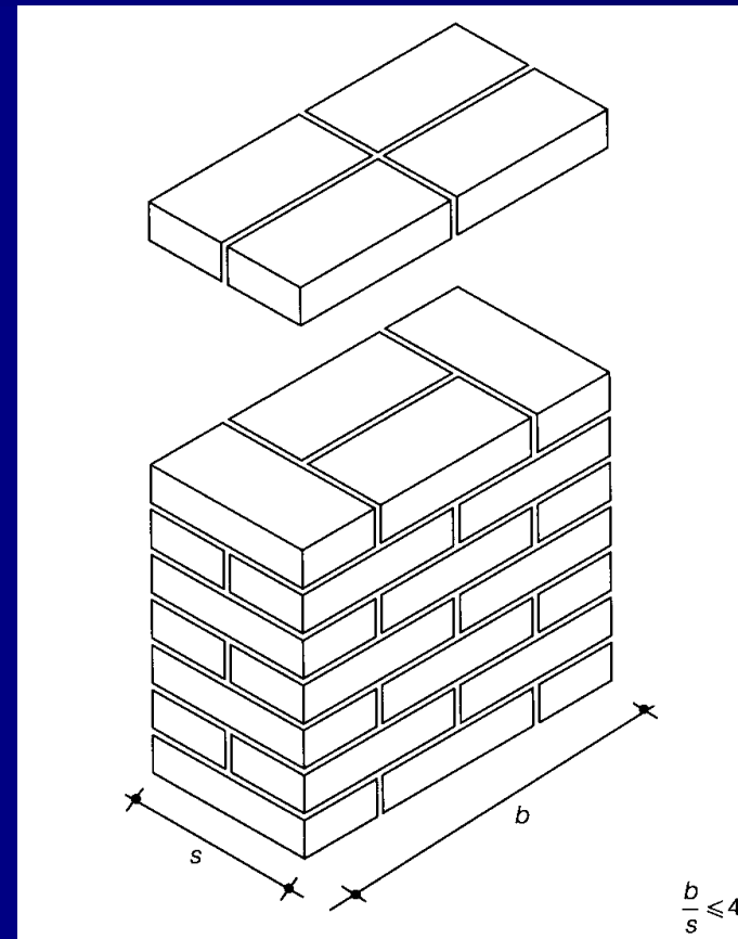
Muratura in laterizio con funzione di pilastro. (Immagine tratta da Carbone et al. , op. cit. )
