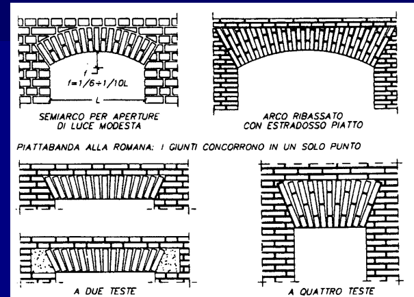
Tipi di piattabanda [Manuale dell'architetto].
