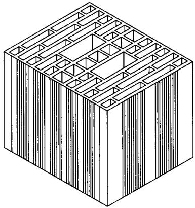
Blocchi in laterizio alleggerito. (Immagini tratte da Carbone et al. , op. cit. )
