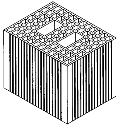
Blocchi in laterizio alleggerito. (Immagini tratte da Carbone et al. , op. cit. )
