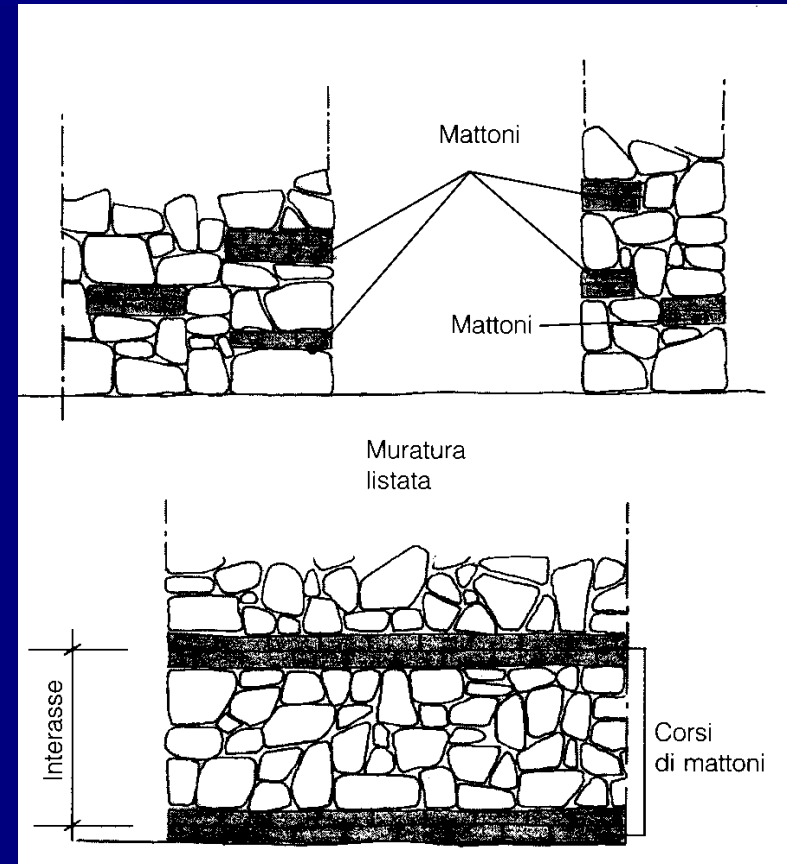
Murature miste in pietra e mattoni. (Immagine tratta da Carbone et al. , op. cit. )
