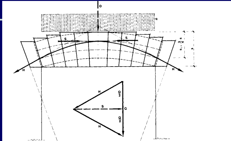
Curva delle pressioni della piattabanda [Alasia, Corso di Costruzioni, SEI].
