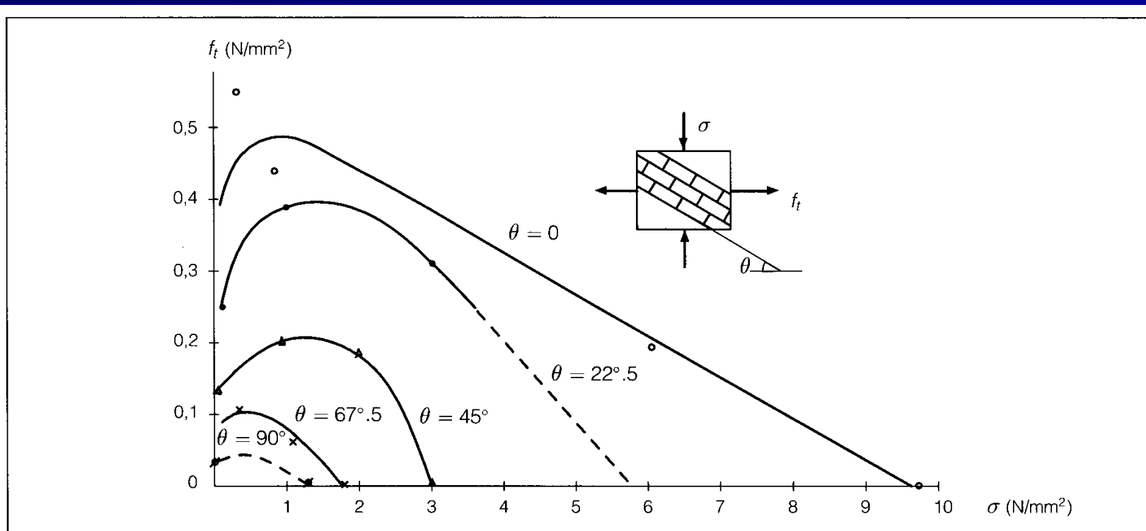
Curve di crisi di pannelli di muratura in regime biassiale per diverse orientazioni dei giunti.
