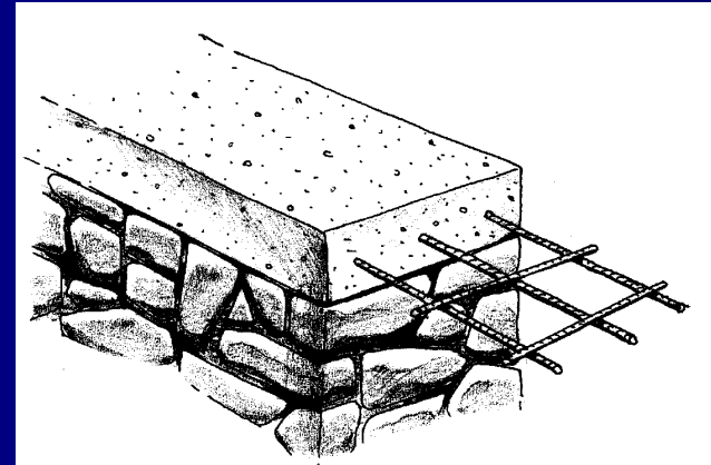
Muratura in pietra con cordoli in c.a.
