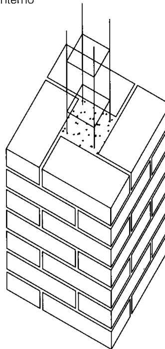
Pilastro in muratura con pilastroino in c.a. all'interno
