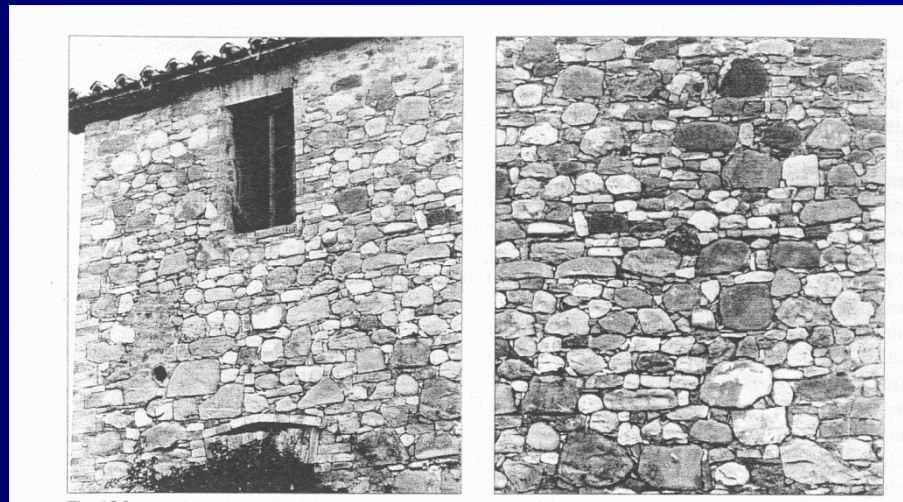
Costruzioni in muratura in pietra naturale. (Immagine tratta da Boscotrecase et al. , op. cit. )
