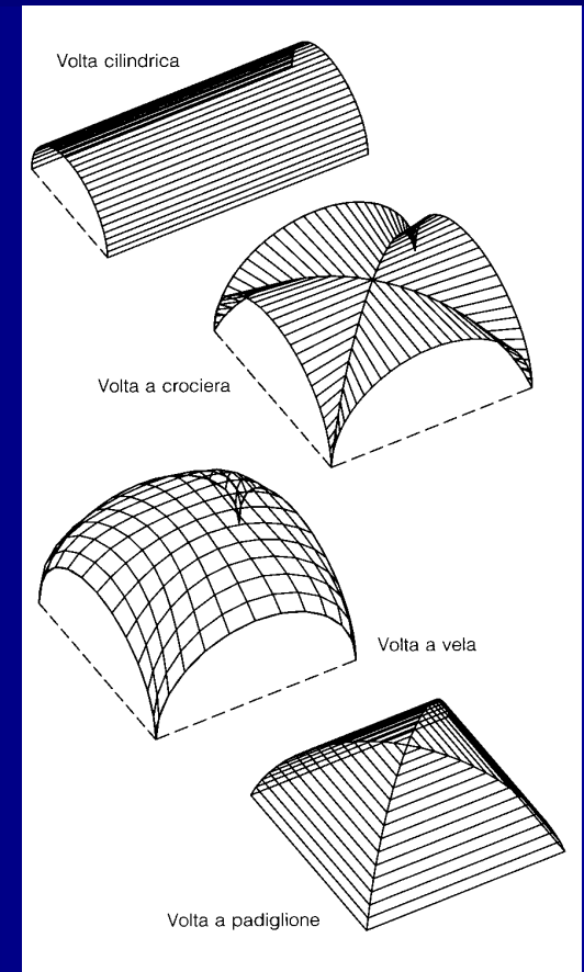
Tipologie di volte.
