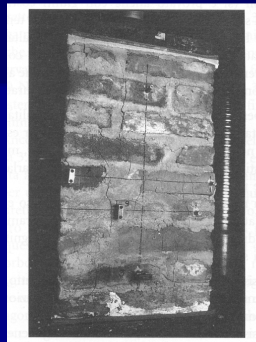
Fessurazioni in un elemento compresso di muratura.
