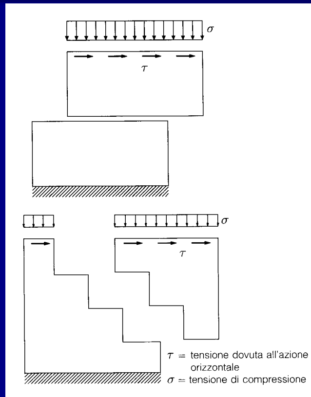
Rottura per scorrimento nei giunti orizzontali. (Immagine tratta da Carbone et al. , op. cit. )
