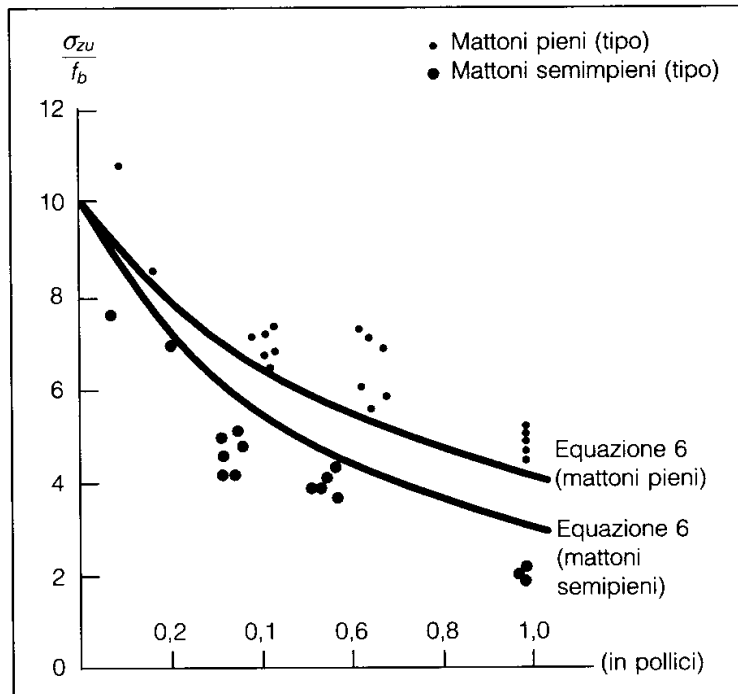
Influenza del rapporto spessore del giunto/altezza del mattone sulla resistenza a compressione della muratura.
