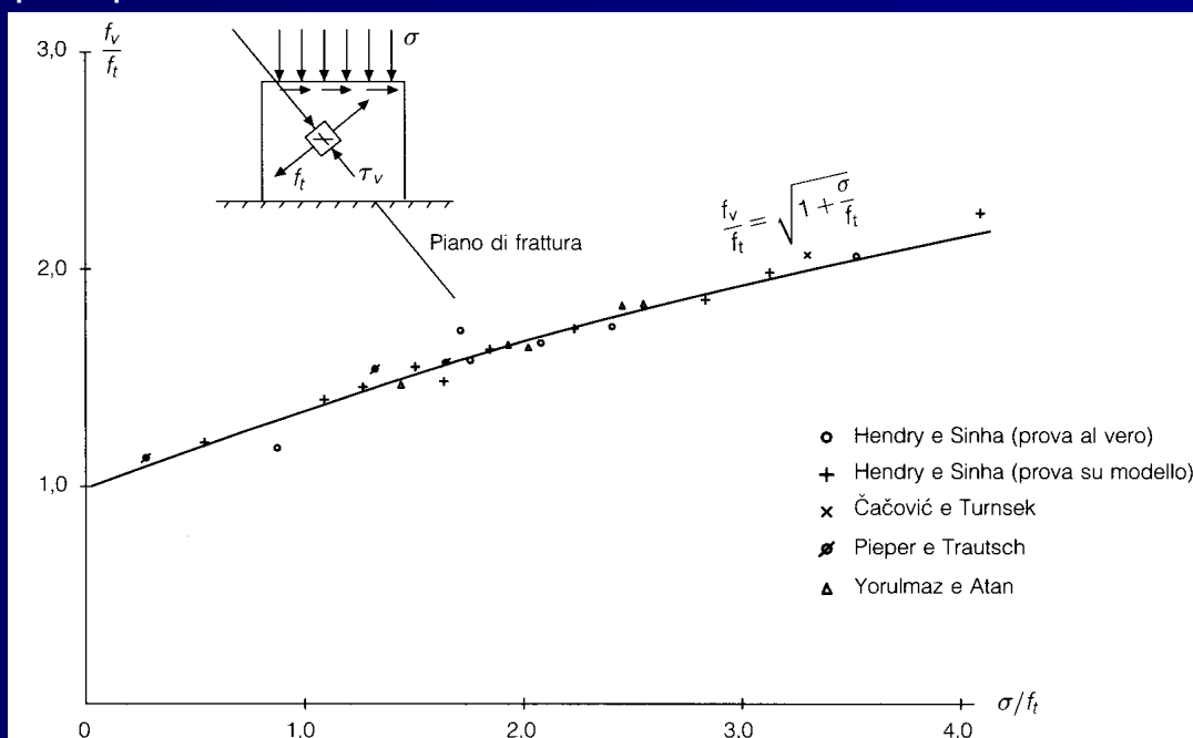
Critero di crisi per taglio-trazione di un pannello in muratura. Diagramma adimensionale della tensione tangenziale media in funzione della compressione applicata. (Immagini tratte da Carbone et al. , op. cit. )
