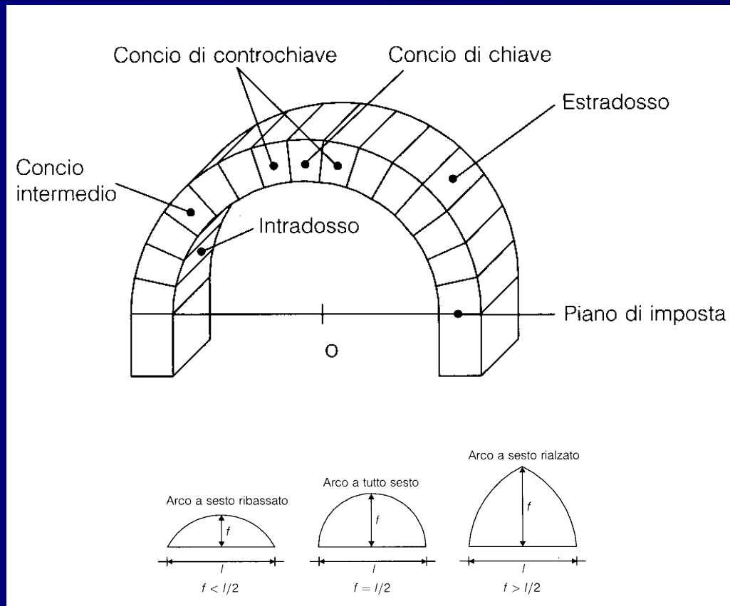
Terminologia degli elementi costitutivi di un arco e tipologie di archi. (Immagine tratta da Carbone et al. , op. cit. )
