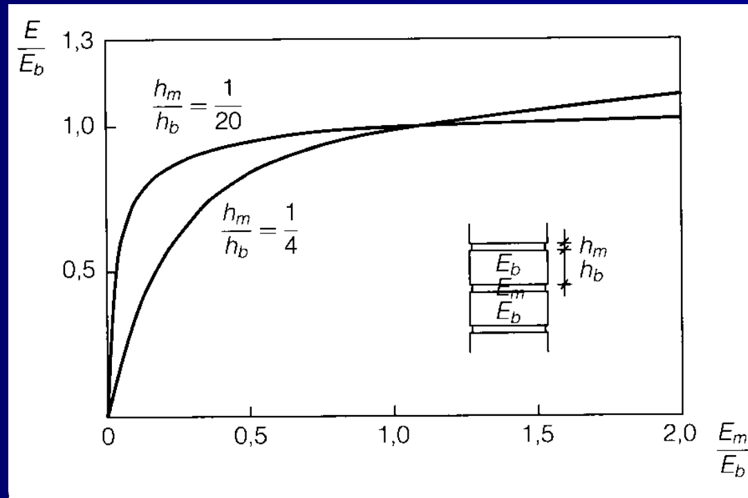
Modulo elastico della muratura, E , in funzione del modulo elastico della malta, E_m . (Immagine tratta da Carbone et al. , op. cit. )
