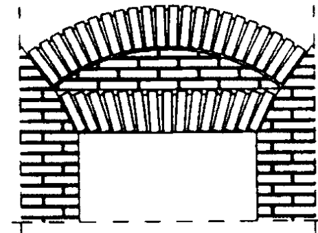
Piattabanda e arco di sordino.
