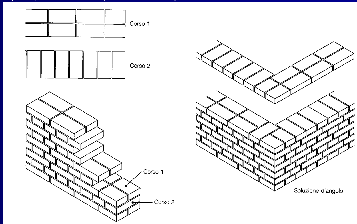
Disposizione a blocco (muratura a due teste).
