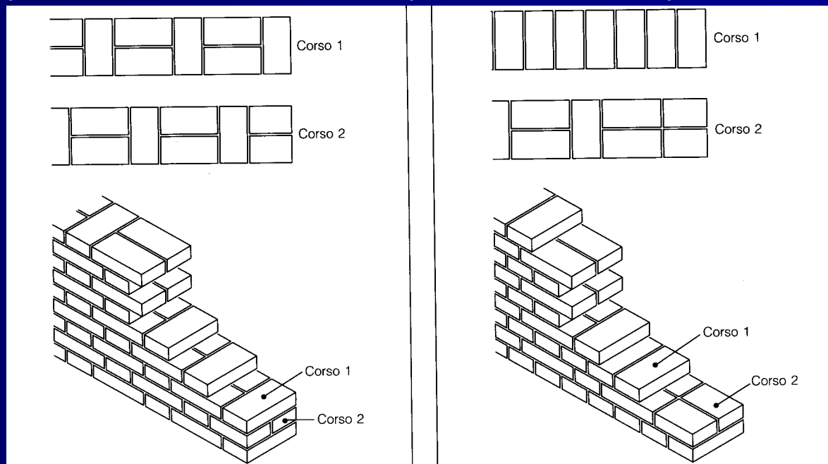
Disposizione gotica e disposizione fiamminga. (Immagine tratta da Carbone et al. , op. cit. )
