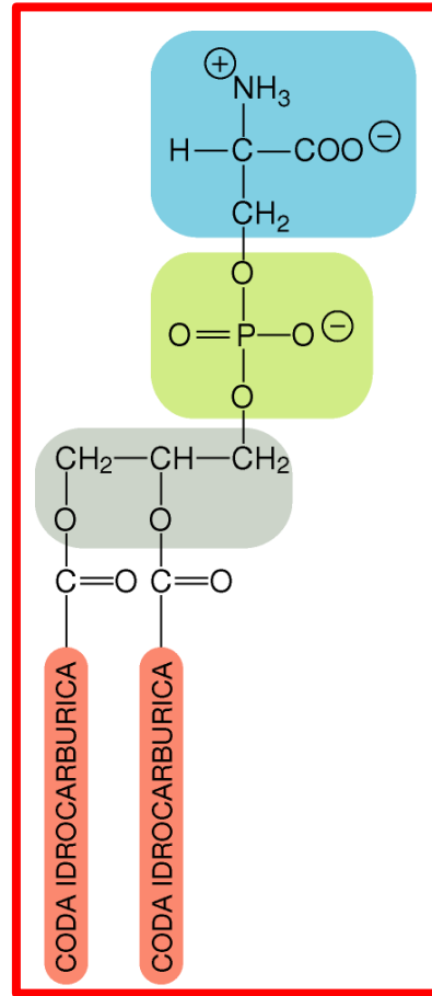
fosfatidilserina (fosfolipide)
