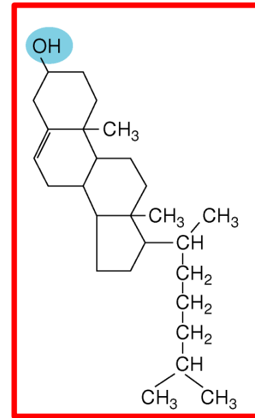
colesterolo (sterolo)
