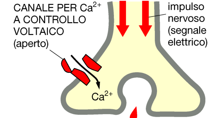
NEUROTERMINALE ATTIVATO
