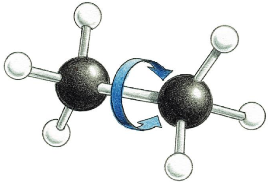
(A) etano
