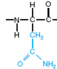
asparagina
