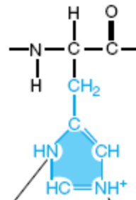
istidina
