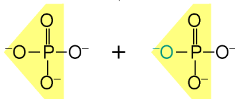
fosfato
