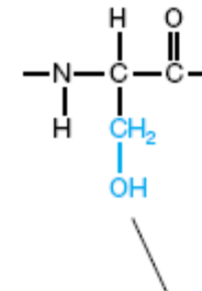
serina
