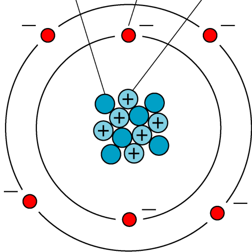
atomo di carbonio
