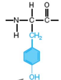
tirosina
