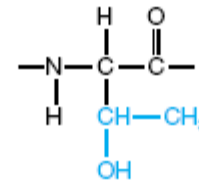
treonina
