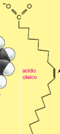
ossatura di carbonio
