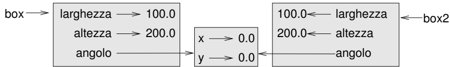
Figura 15.3: Diagramma di oggetto.
