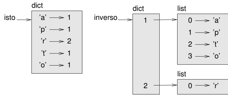
Figura 11.1: Diagramma di stato.
