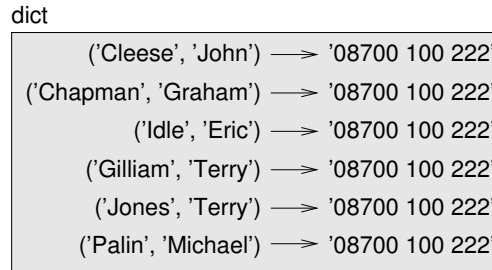
Figura 12.2: Diagramma di stato.
